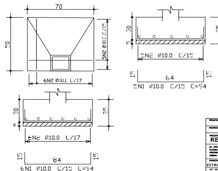
SAPATAS - 90X70 - SP2
