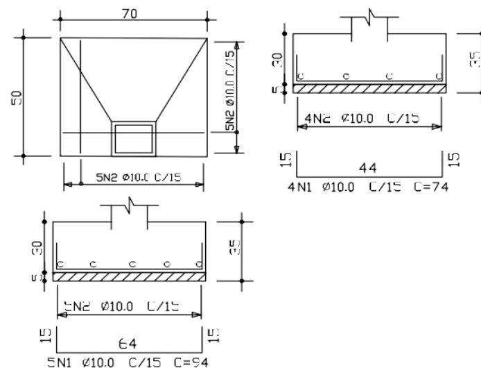
SAPATAS - 70X50 - SP2
