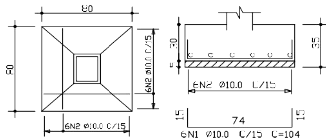
SAPATAS - 80X80 - SP5
