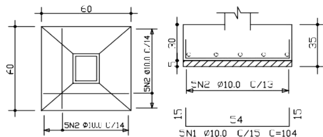
SAPATAS - 60X60 - SP1, SP3 e SP4
